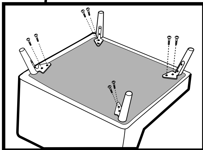
Bolts 24 pc (8 per modul) - 6x30 mm
